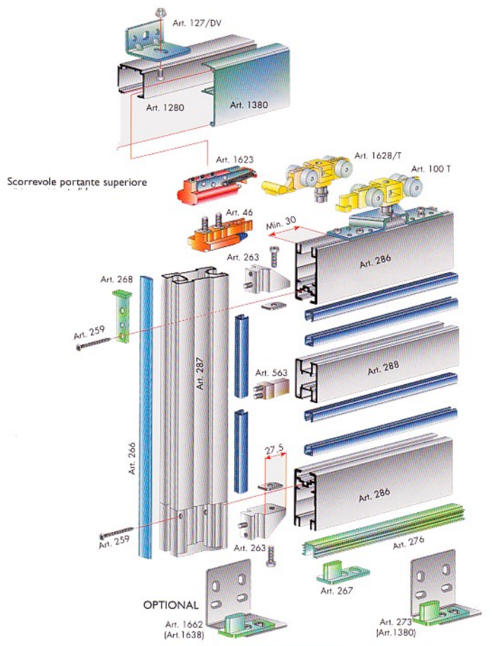
Ternoscorrevoli porta alluminio
